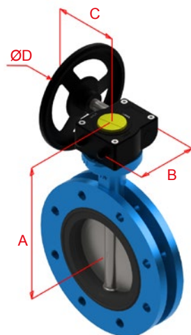
Reductor Worm-gear
